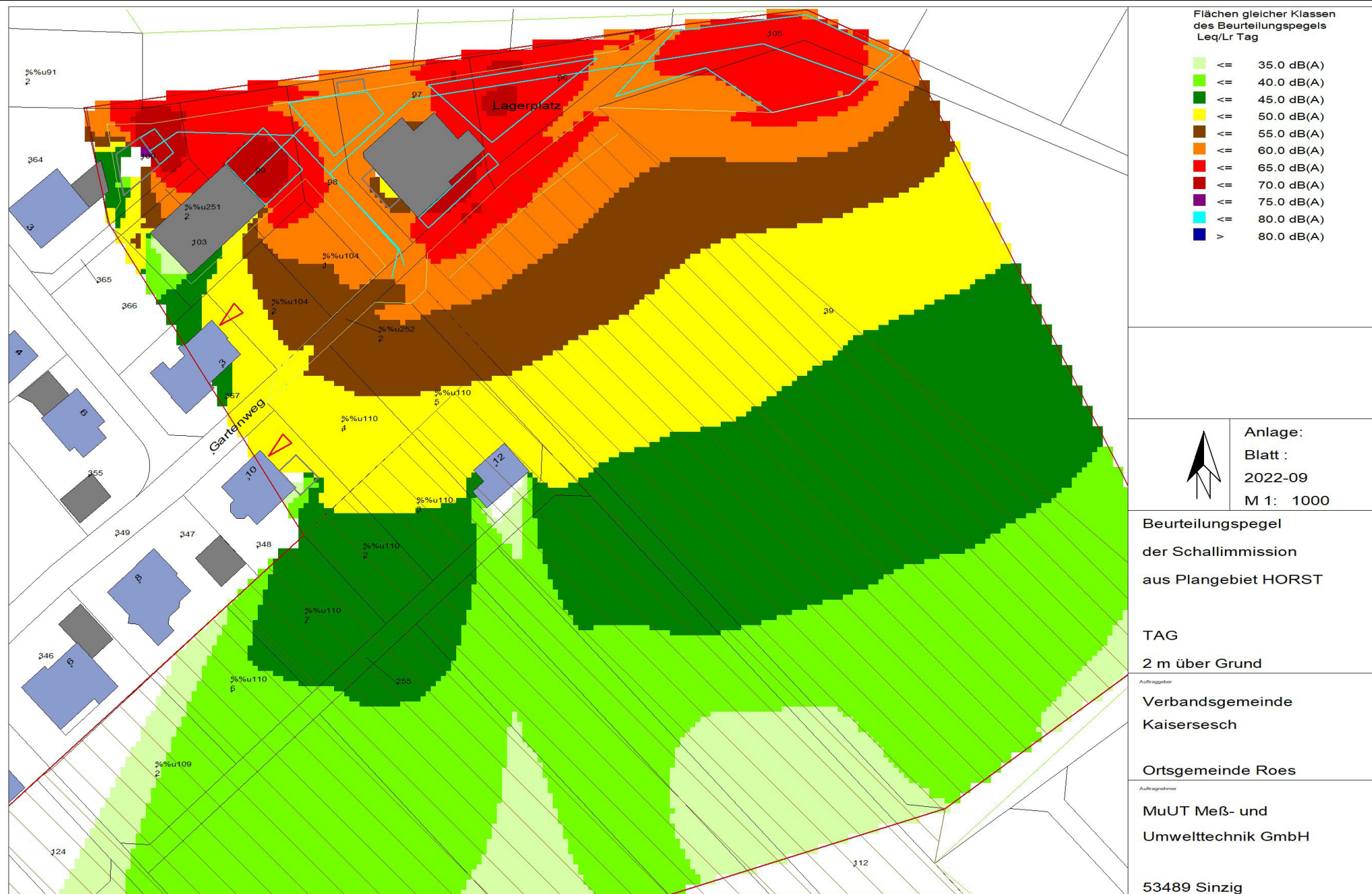
Abb. 10: Beurteilungspegel Gewerbe aus Bebauungsplan Horst, Tageszeit in 2 m Höhe über Grund
