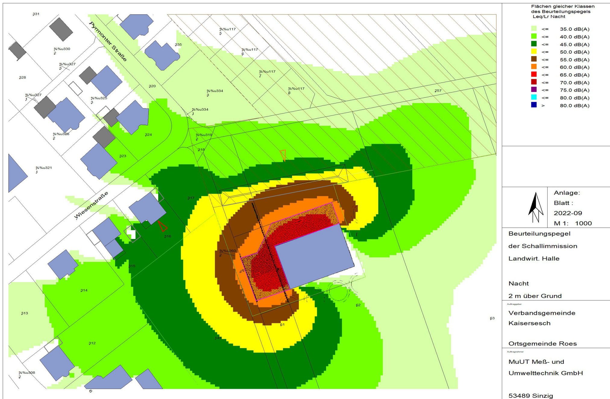
Abb. 7: Beurteilungspegel landwirtschaftliche Halle, ungünstigste Nachtstunde in 2 m Höhe über Grund
