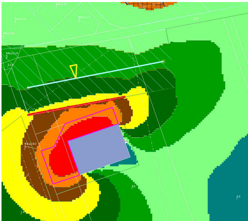
Abb. 2: Schallimmission ungünstigste Nachtstunde in 2 m Höhe über Grund, dargestellt in 5 dB Farbklassen dunkelgrün: Richtwert Mischgebiet 45 dB(A) eingehalten oder unterschritten
