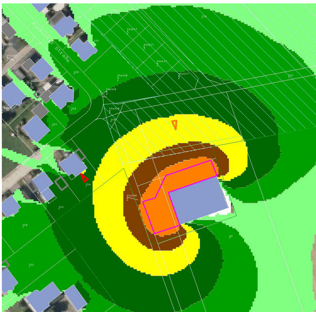
Abb. 5: Beurteilungspegel der Schallimmission nachts, 5 m über Grund, nur An- oder Abfahrt (vgl. Text) ab Dunkelgrün: Richtwert Mischgebiet eingehalten; rotes Dreieck: Bestands- haus Wiesenstraße 8
